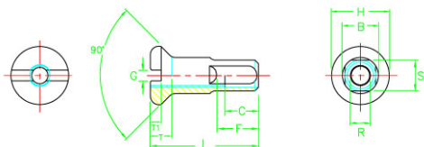
Rysunek techniczny nakrętki szprychy L = długość nypla
