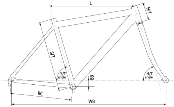
HARDTAIL: Kellys Protec 6061 - SG (Sport Geometry)
